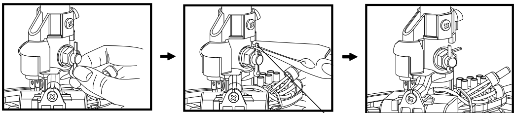
Cotter Pin is bent / 開口銷被折彎 / Chốt hãm nêm được bẻ gấp xuống
